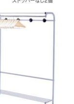
11-559-20 コートハンガー B(グレー) ¥ 56,300 (W1,200・D370・H1,600) ●スチール角パイプ ●メラミン焼付塗装 ●ハンガー10本付
