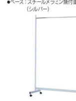
11-559-25 コートハンガー ¥ 42,300 (W1,200・D500・H1,600) ●本体：スチール(46×20mmダ円パイプ)メラミン焼付塗装 ●ハンガーパイプ：スチール(φ25.4mm)クロームメッキ ●φ40mm双輪キャスター付
