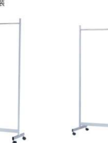
11-559-26 コートハンガー ¥ 44,700 (W1,600・D500・H1,600) ●本体：スチール(46×20mmダ円パイプ)メラミン焼付塗装 ●ハンガーパイプ：スチール(φ25.4mm)クロームメッキ ●φ40mm双輪キャスター付
