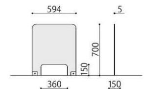
VCH-AR
