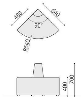
RO-SOR90
