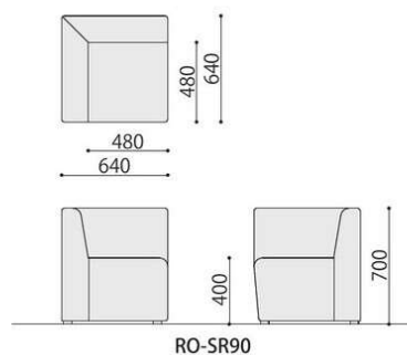
RO-SR90
