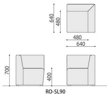
RO-SL90
