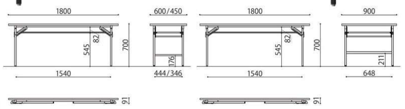
VKT-1860B-1845B
