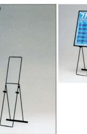
11-403-28 ¥ 27,000 (面板寸法：W297・H420) (外寸法：W312・H1,307・D300) (有効画面寸法：284×407) 重量：5.1kg
